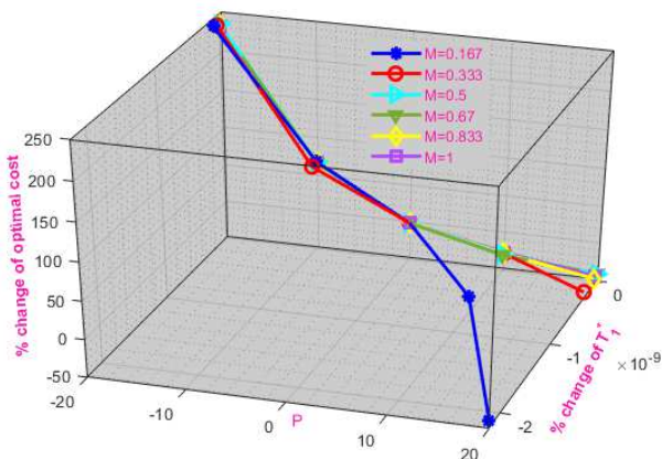
(a) Parameter p
