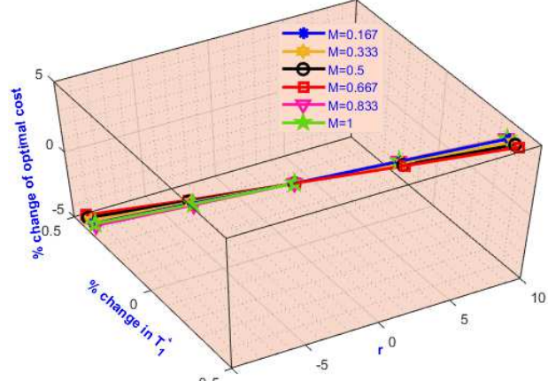
(d) Parameter r
