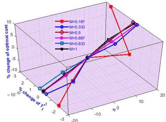
(b) Parameter \eta
