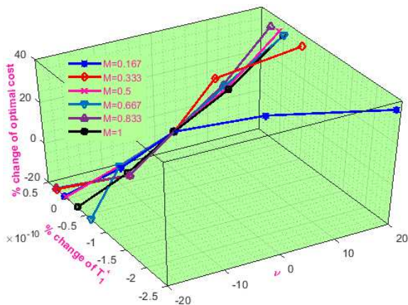
(c) Parameter \nu
